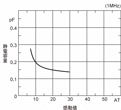
接点間静電容量
